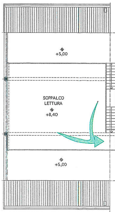
PIANTA PIANO QUOTA +8,40
